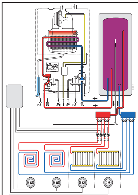
Installatieschema MegaDens HR-ketel i.c.m. Energie Visie Vat
